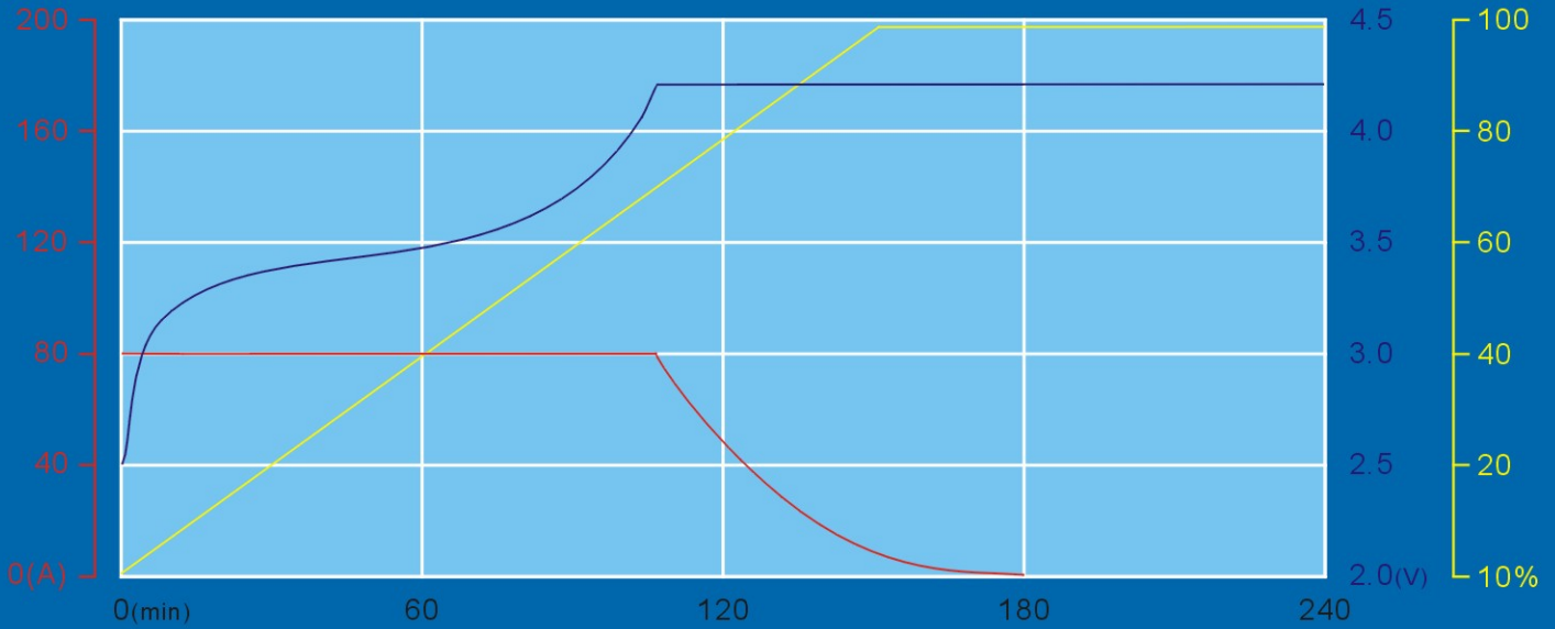
TS-LFP160AHA在25°C環境下的充電特性 TS-LFP160AHA CHARGE AT TEMPERATURE OF 25°C
