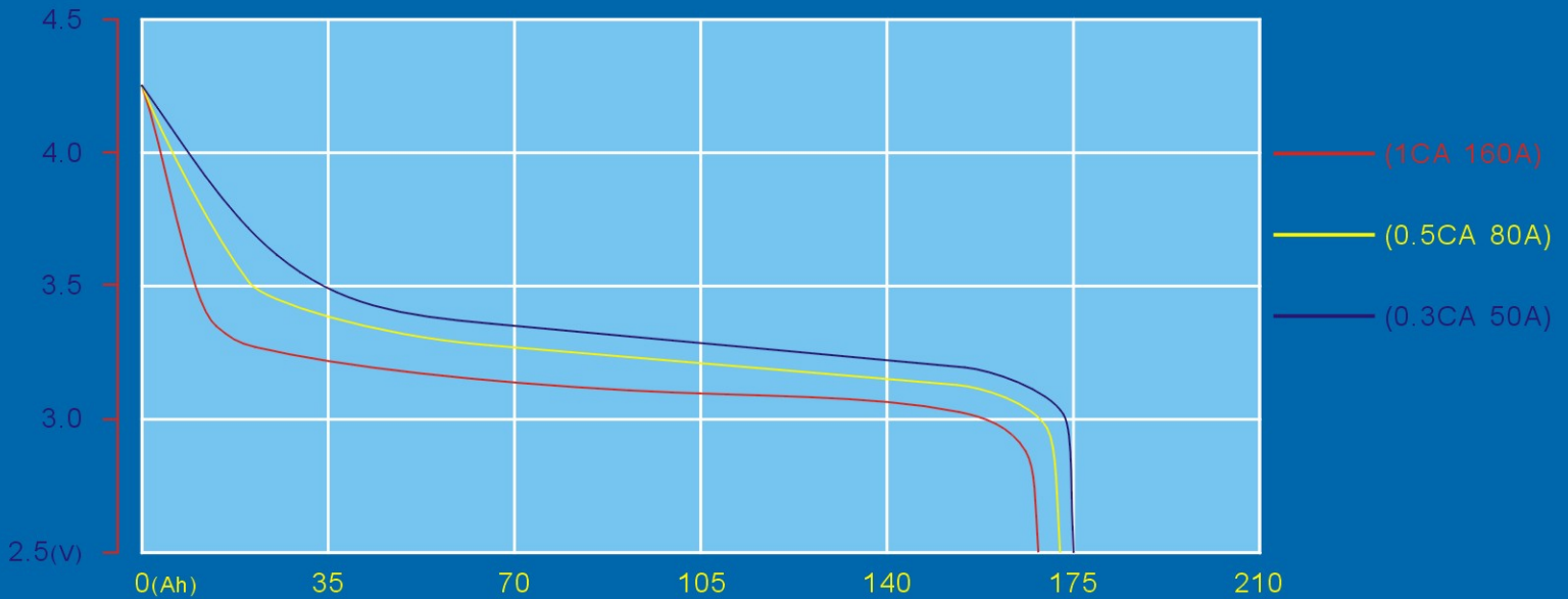
TS-LFP160AHA在25°C環境下的放電特性 TS-LFP160AHA DISCHARGE AT TEMPERATURE OF 25°C
