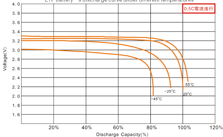
不同環境溫度下LFP類電池的放電特性曲線 LYP battery's discharge curve under different temperatures
